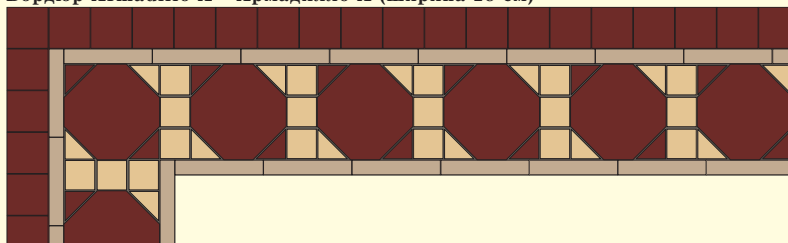
Бордюр Armadillo A - Армадилло А (ширина 28 см)
